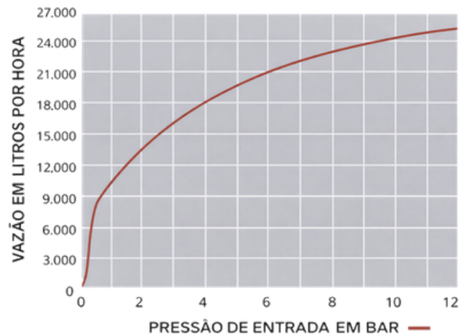
CURVA DE VAZÃO E PRESSÃO DA BOIA
